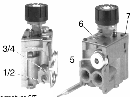
Plynová armatura SIT
