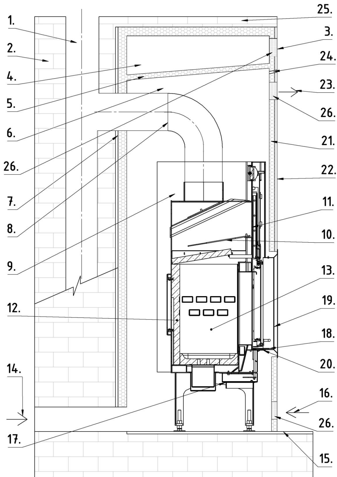
Obr. 4. Řez typickou obezdívkou.
