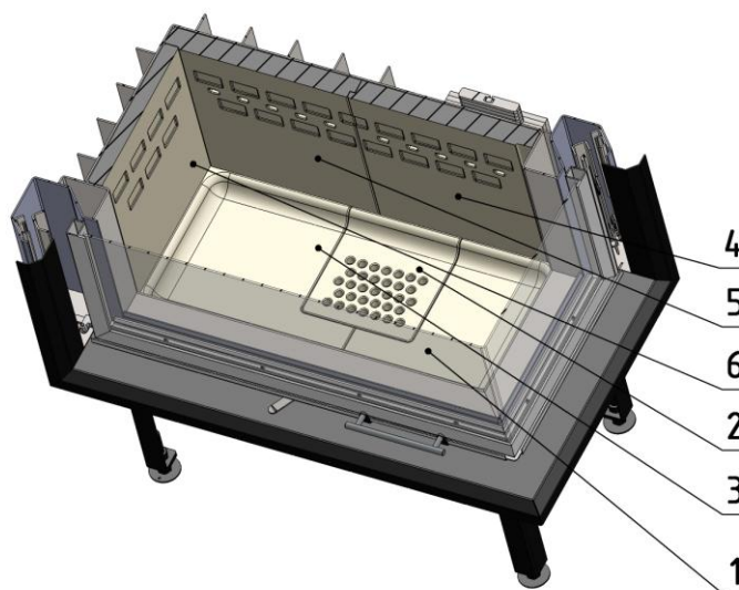
Obr. č. 3A. Pohled na sestavu vyložení topeniště – rohová varianta.
