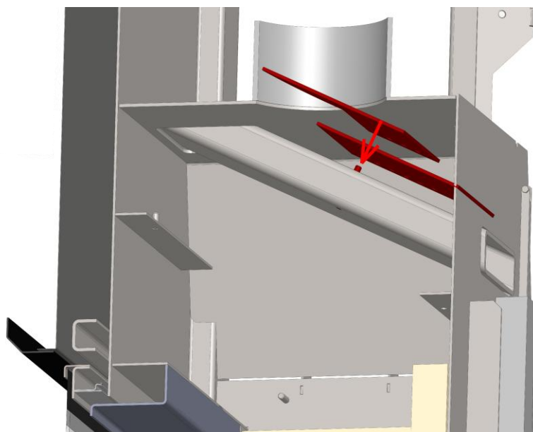
Obr. č. 2A. Montáž deflektorů výměníku.
