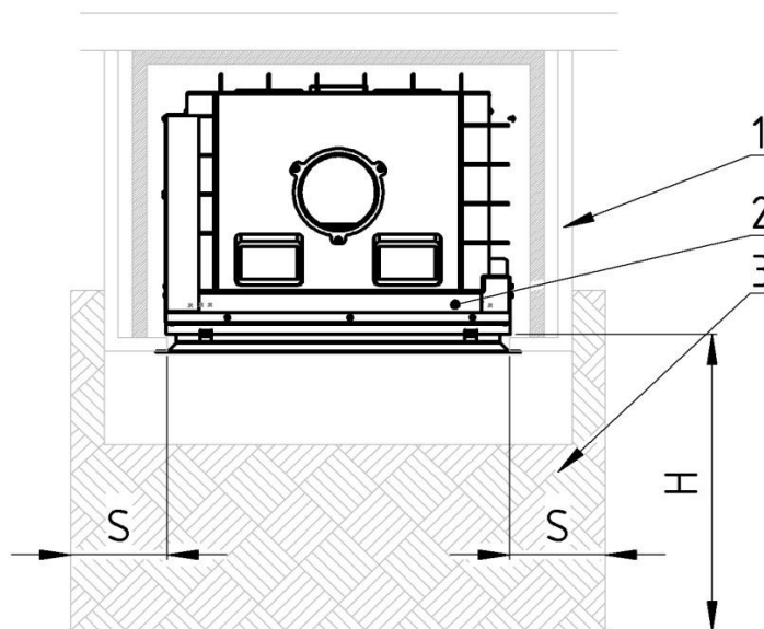
Obr. 7. Nutné přesahy nehořlavé podklady pro instalaci vložky.
