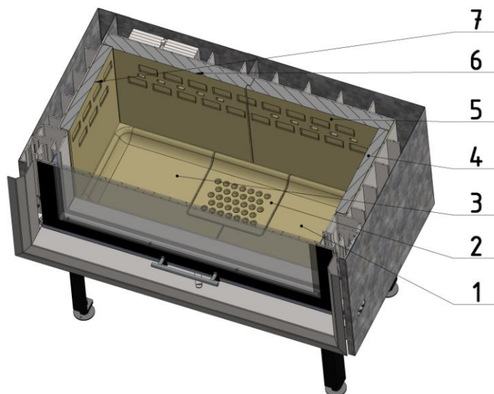
Obr. č. 3B. Pohled na sestavu vyložení topeniště – čelní varianta.
