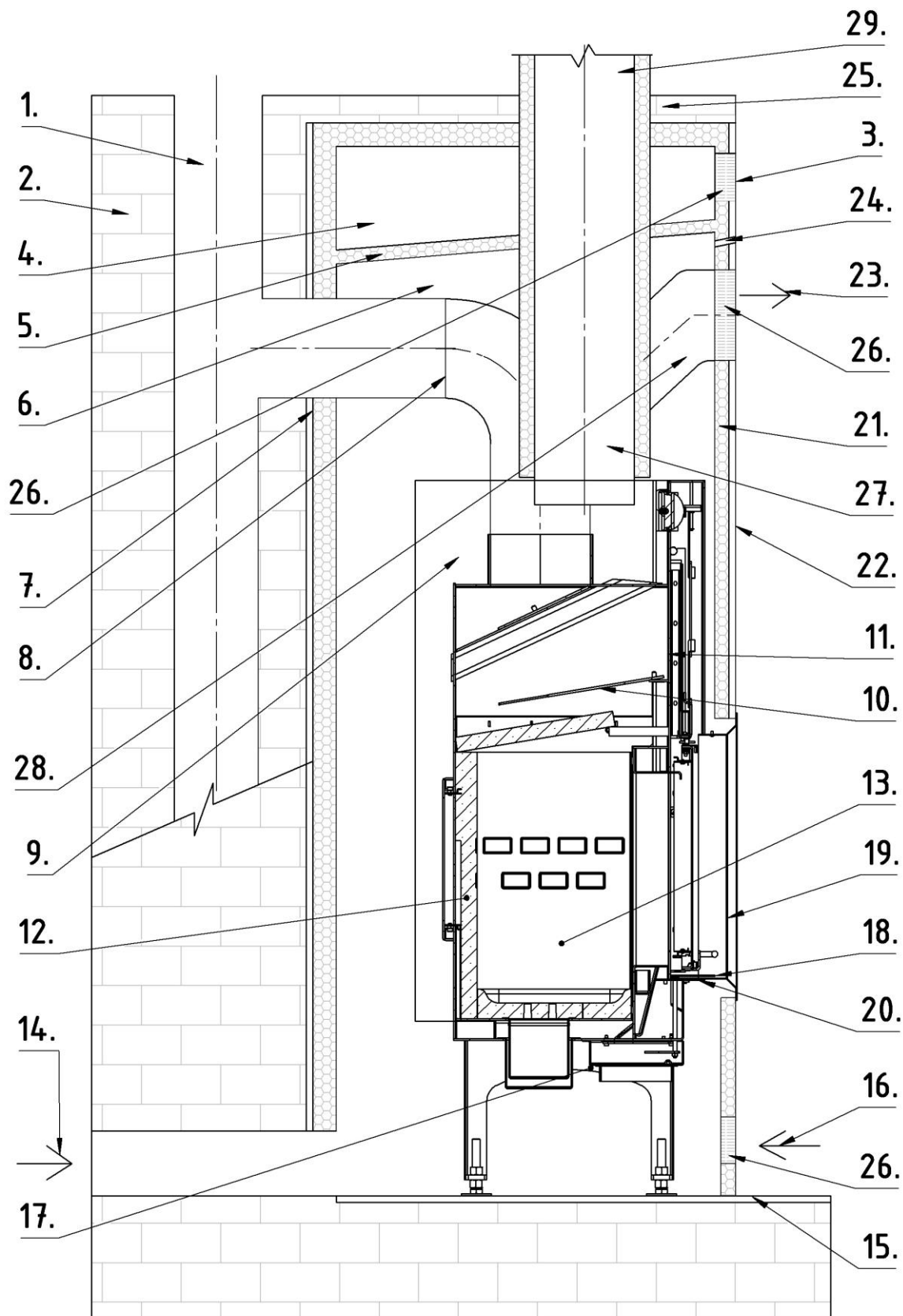
Obr. 5. Řez typickou obezdívkou – instalace včetně teplovzdušného výměníku.
