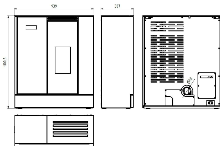
Рис. № 1 Главные размеры
