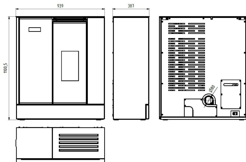
Obr. č. 1 Hlavné rozmery
