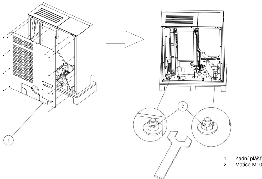
Obr. č. 3 Demontáž krbových kamen z palety
