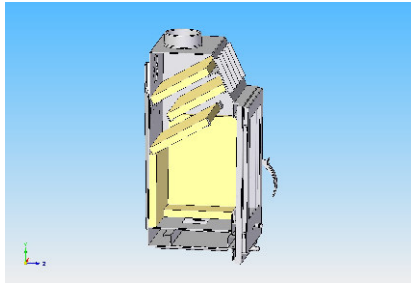
7. vložení náhradního dílu ND-13.3
