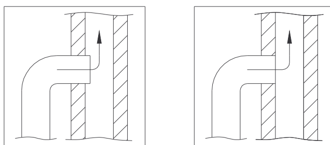
nesprávně Připojení na komín správně obr.č.1
