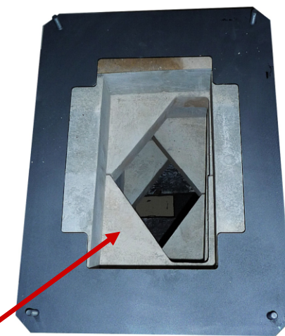
akumulační výplň
